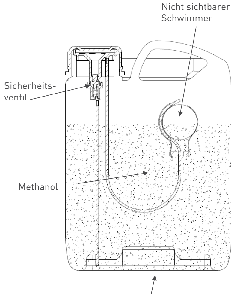
Kanister UN-zertifiziert
